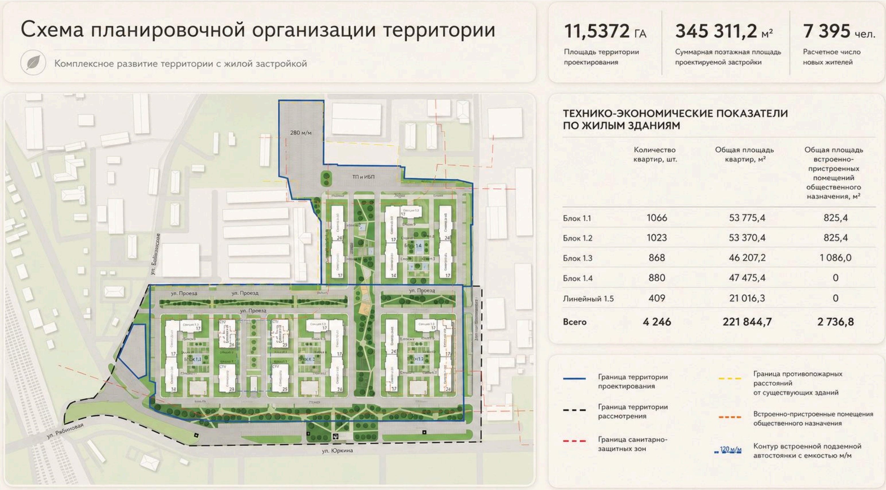
Схема планировочной организации территории
